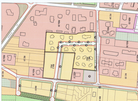
ESTRATTO DI PRGC CON INSERIMENTO DELL'INTERVENTO IN PROGETTO Scala 1:2.000
