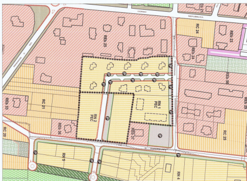
ESTRATTO DI PROGETTO Scala 1:2.000
